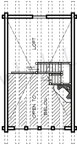
LOFT 180 SQ FT
